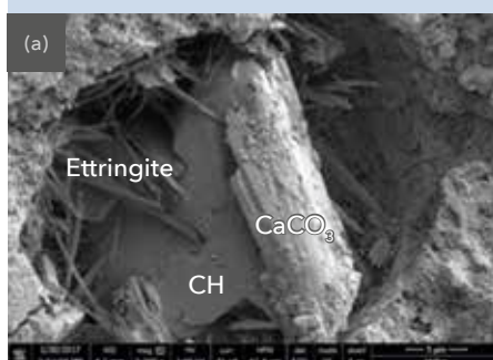
Images MEB de pores bouchés par des cristaux dans un béton réalisé avec VANDEX AM 10 (a) ou VANDEX SUPER (b)
